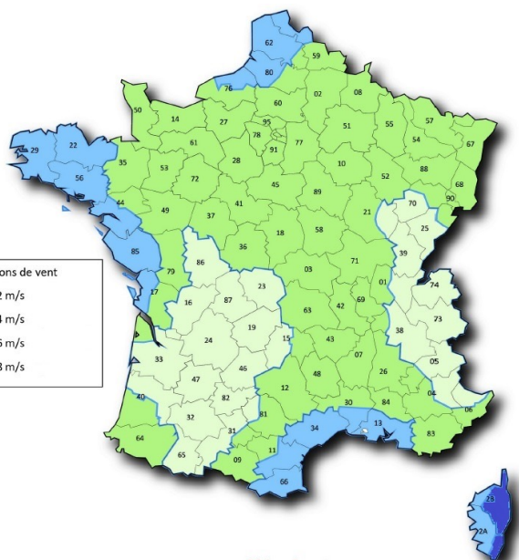
Régions de vent Annexe Nationale de l'EN 1991-1-4
